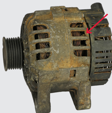
Estátor quemado
