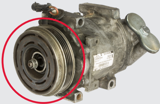
Moyeu manquant
