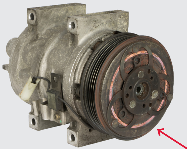
Le moyeu ne peut pas tourner et l'embrayage est brûlé
