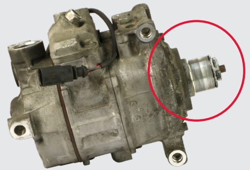
Poulie manquante
