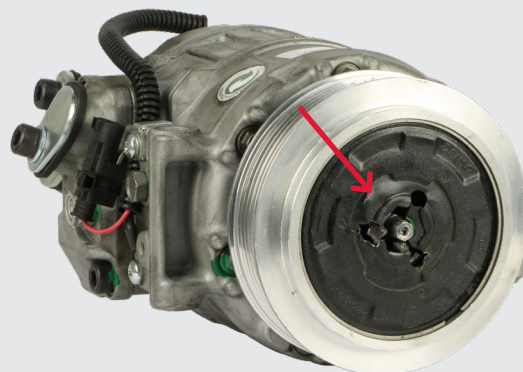
Moyeu cassé
